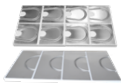
Schets van breuklijnen VA 12,5
